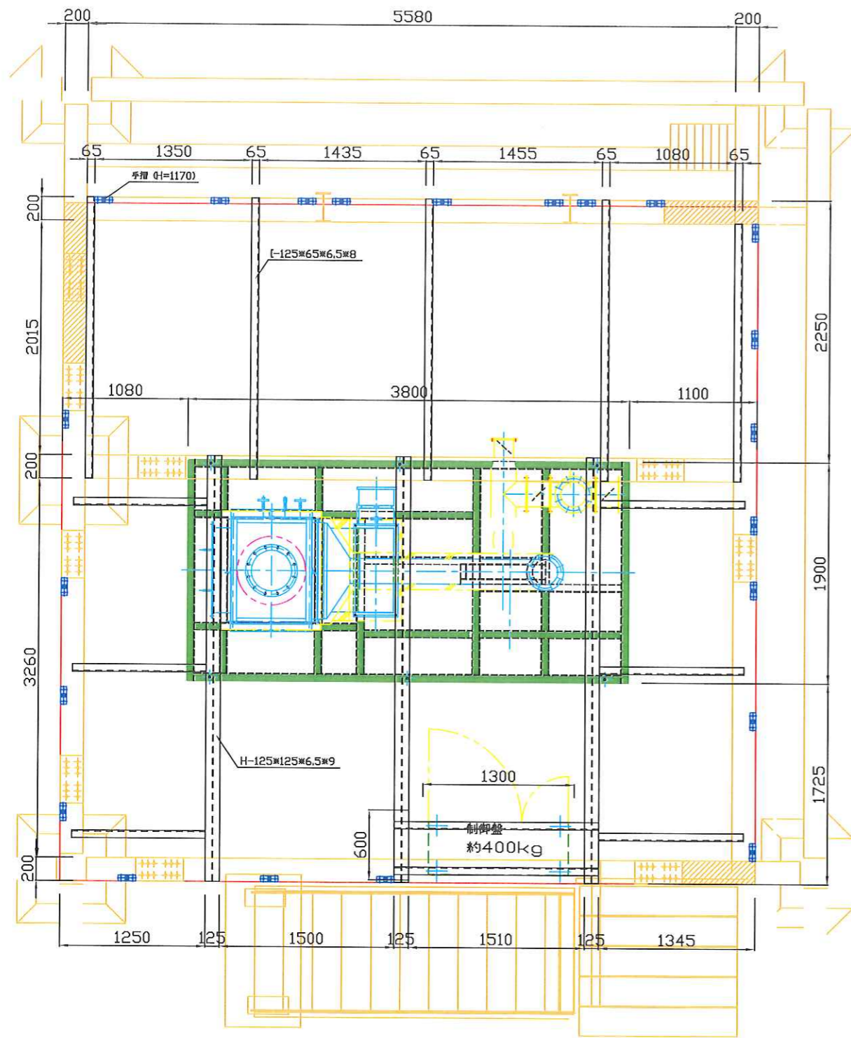
架台図
