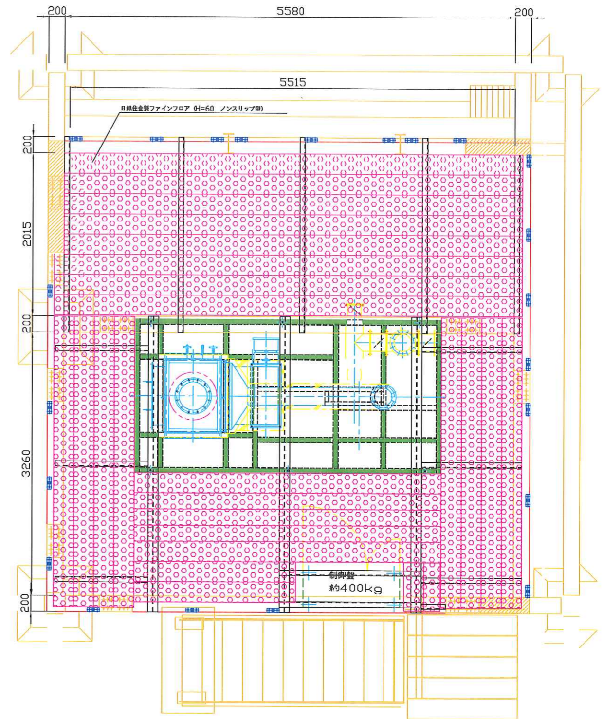
全体図
